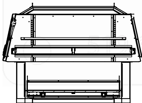
SECTION AB-AB SCALE 1 : 30
